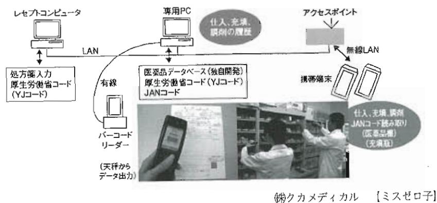
第2図 調剤薬局内 ミスゼロ子システム構成
